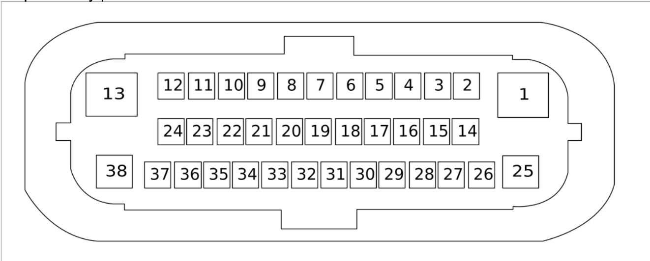
Сторона разъема
